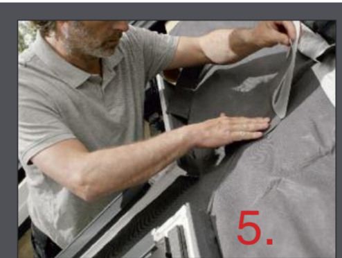
Mit dem im Lieferumfang enthaltenen Klebeband lassen sich die übereinandergelegten, glatten Schürzen ganz einfach und sicher abdichten.
